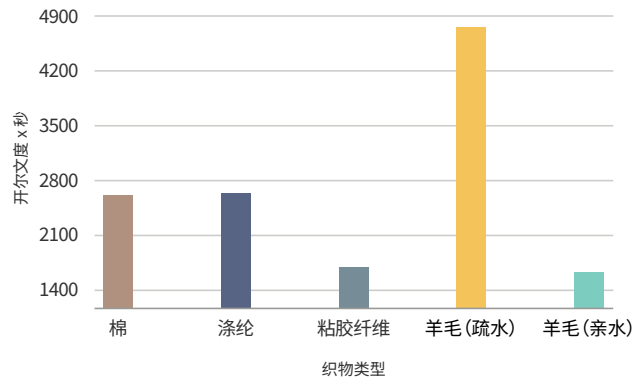
图3 冷却阶段的热量滞留
