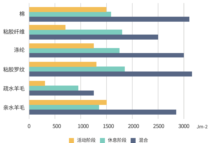
图7 30分钟活动和30分钟休息阶段的能量曲线
